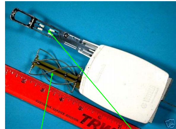
GPS Antenna
